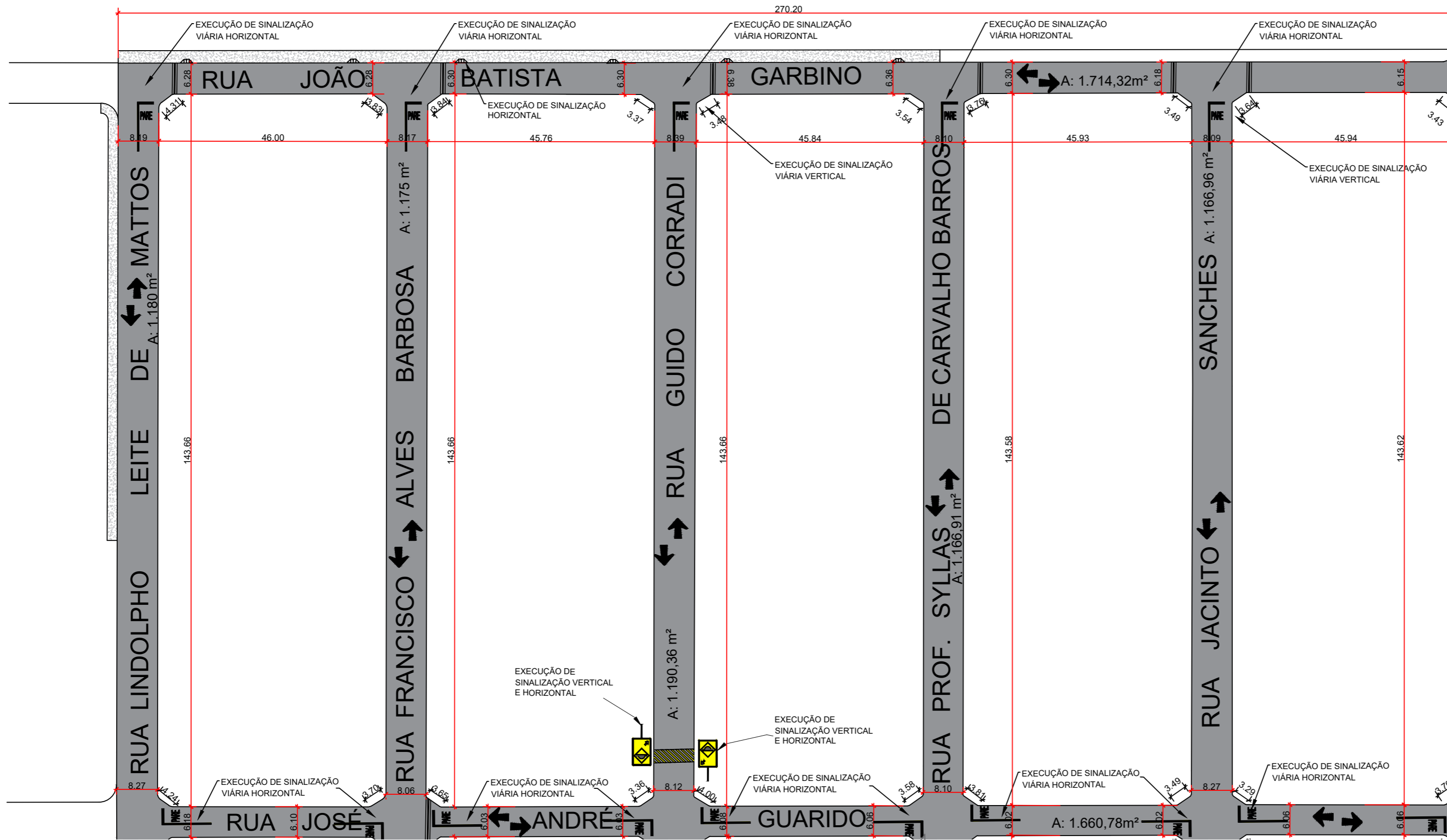
PLANTA - RECAPEAMENTO ASFÁLTICO E SINALIZAÇÃO DE TRÂNSITO - (-22.449753359368668, -48.990331316498654) - PARTE 1/3 - Área = 9.254,33 m 2 ESCALA: 1/750
