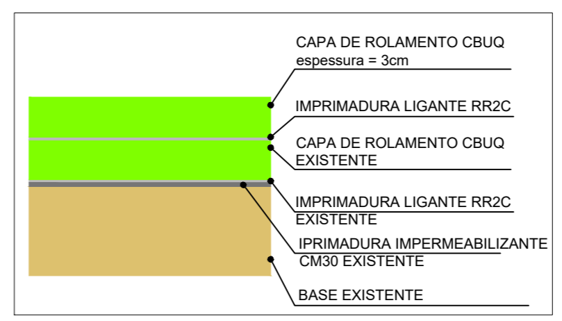
SEM ESCALA DETALHE RECAPE
