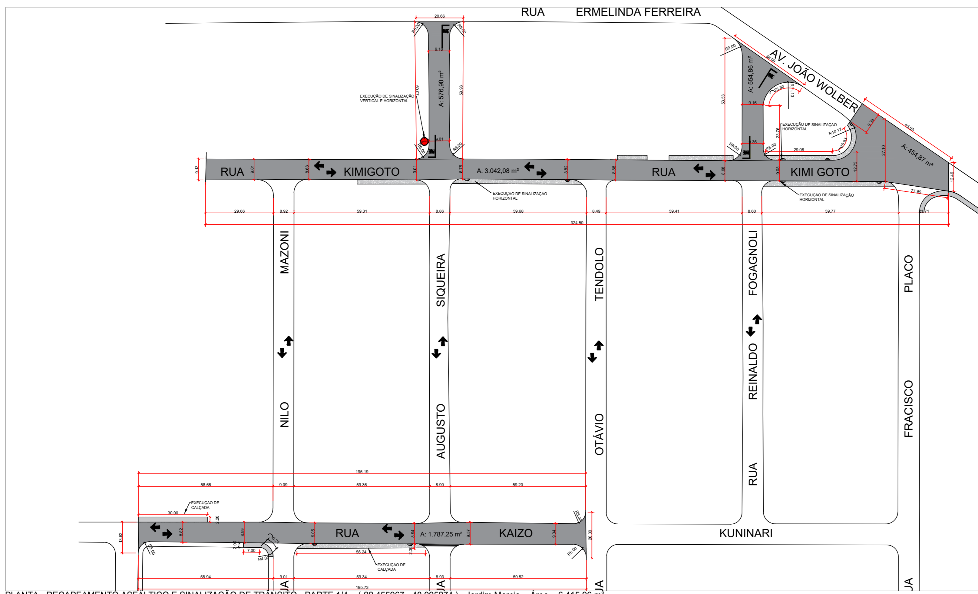
PLANTA - RECAPEAMENTO ASFÁLTICO E SINALIZAÇÃO DE TRÁNSITO - PARTE 1/4 - (-22.455967, -48.995274) - Jardim Marcia - Área = 6.415,96 m 2 ESCALA: 1/1000
