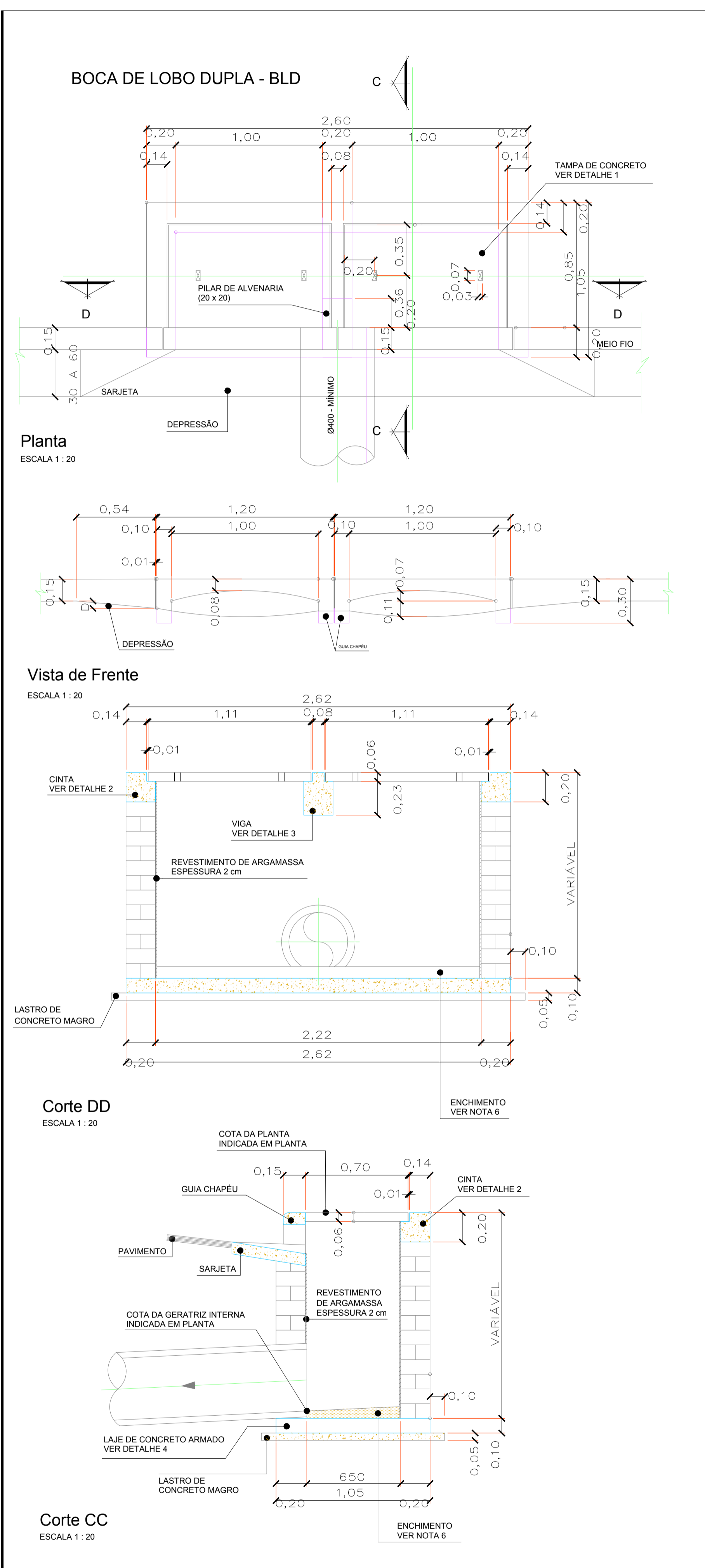
DETALHE BOCAS DE LOBO ESCALA: 1:20
