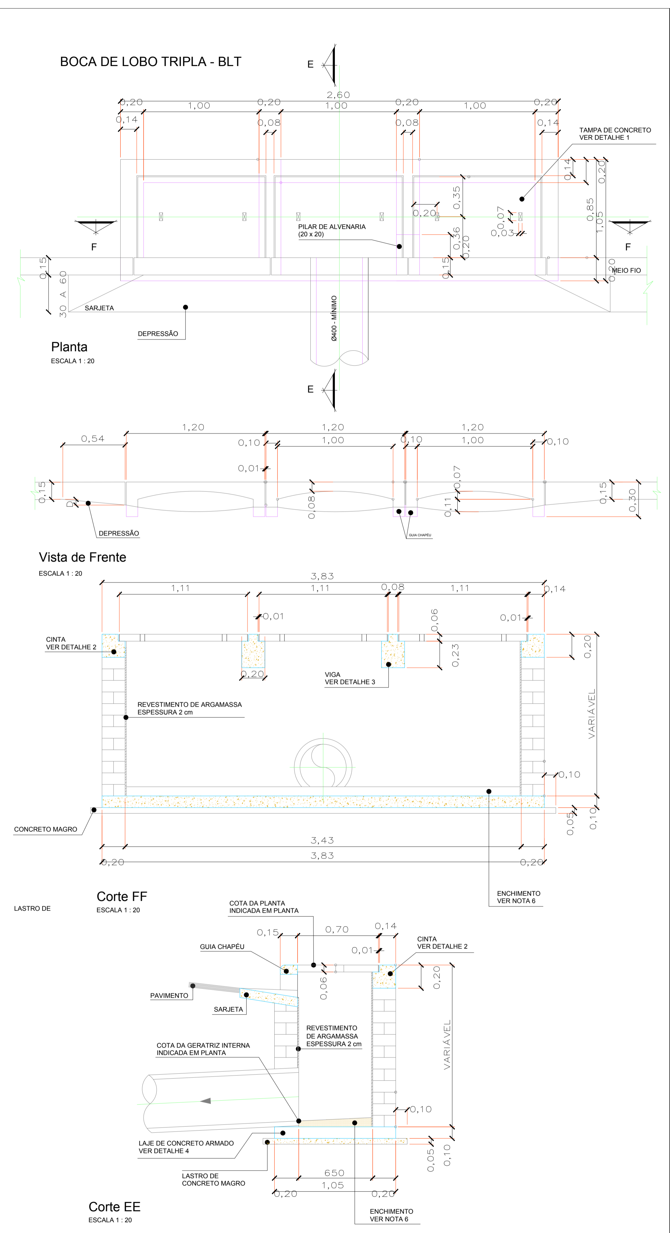
DETALHE BOCAS DE LOBO ESCALA: 1:20
