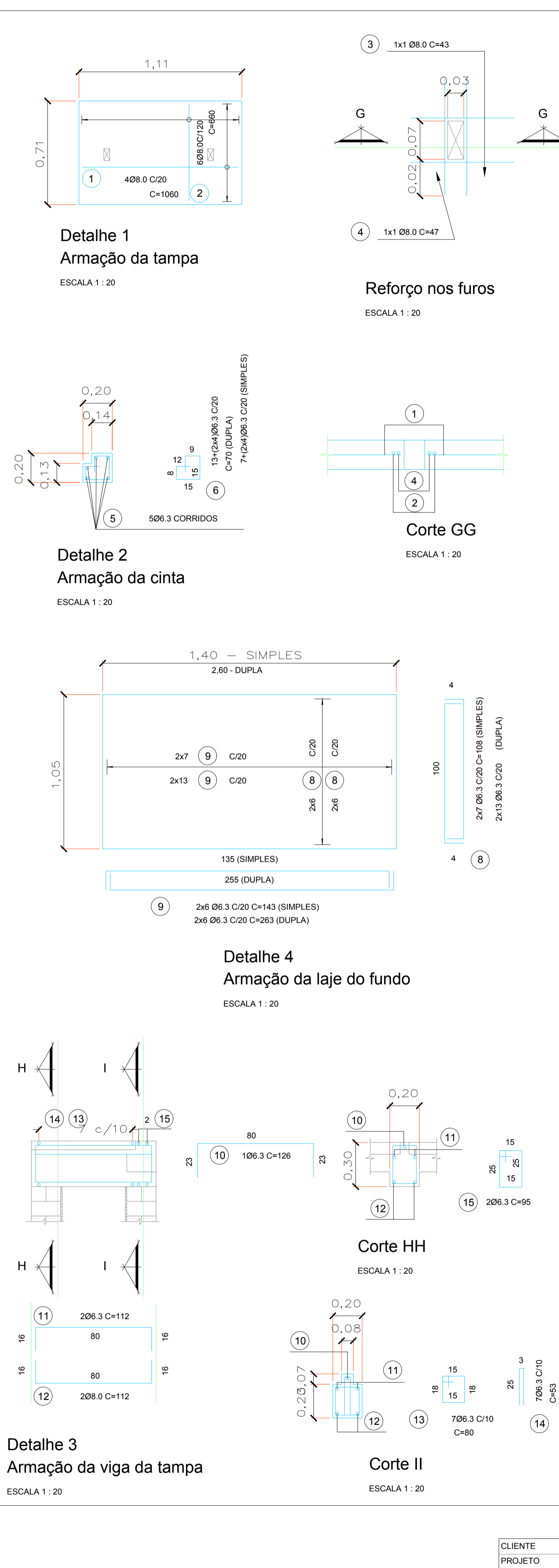
DETALHE BOCAS DE LOBO ESCALA: 1:20
