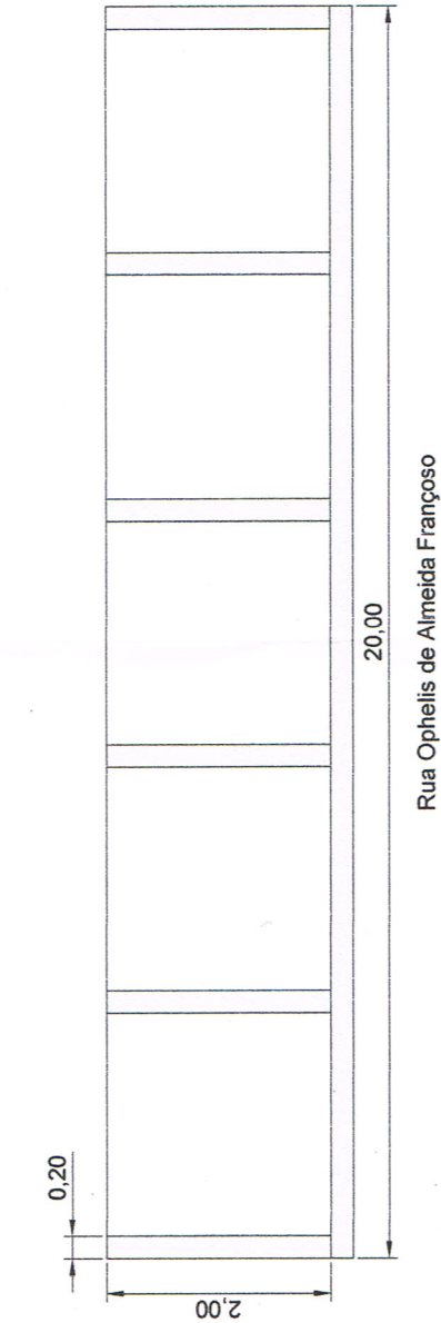
PLANTA: MURO DE ARRIMO
