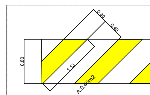
DETALHE SINALIZAÇÃO LOMBADA ESCALA: S/ESCA
