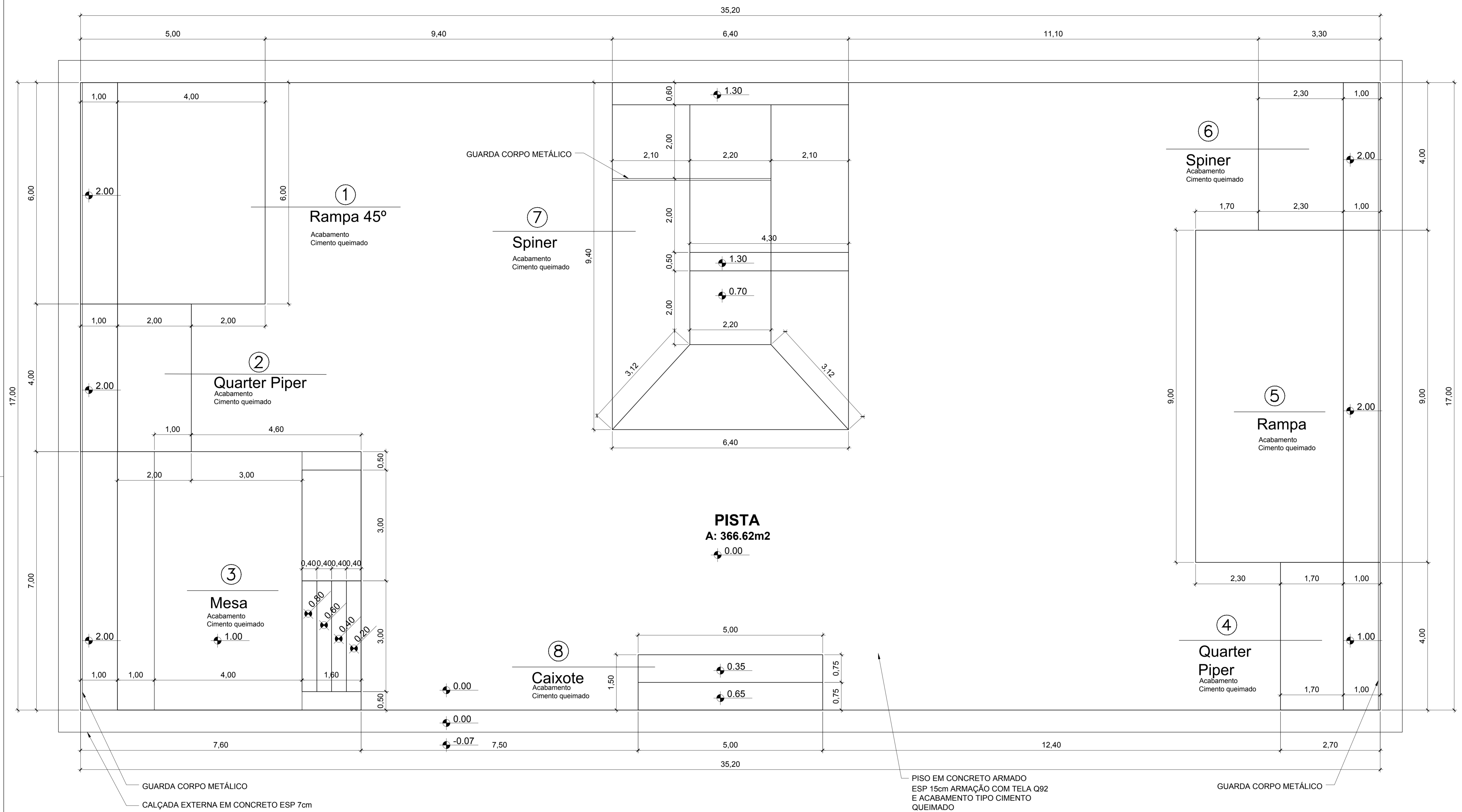
PLANTA ESCALA: 1/50
