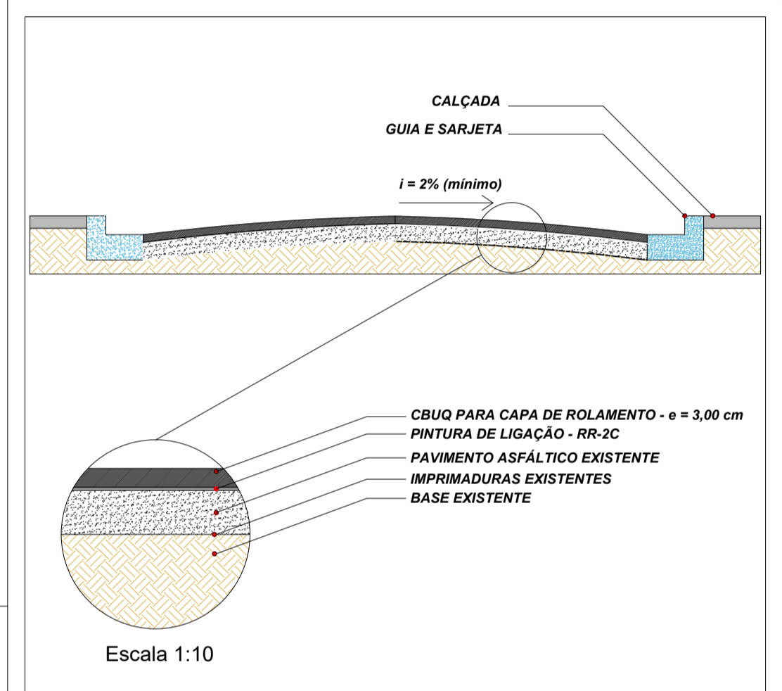
DETALHE CAMADAS DO RECAPE ASFÁLTICO Sem escala
