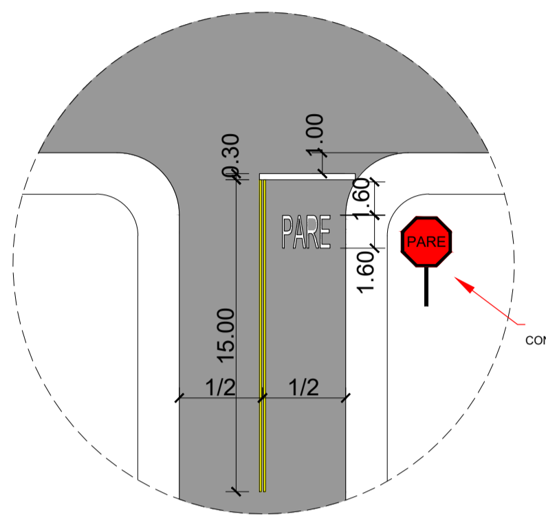
DETALHE SINALIZAÇÕES HORIZENTAIS ESCALA: 1:25
