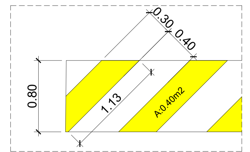
DETALHE SINALIZAÇÕES HORIZENTAIS - LOMBADA ESCALA: 1:25
