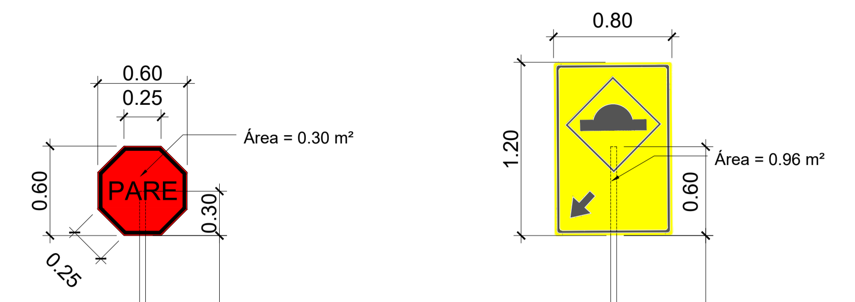
DETALHE SINALIZAÇÕES VERTICAIS ESCALA: 1:25
