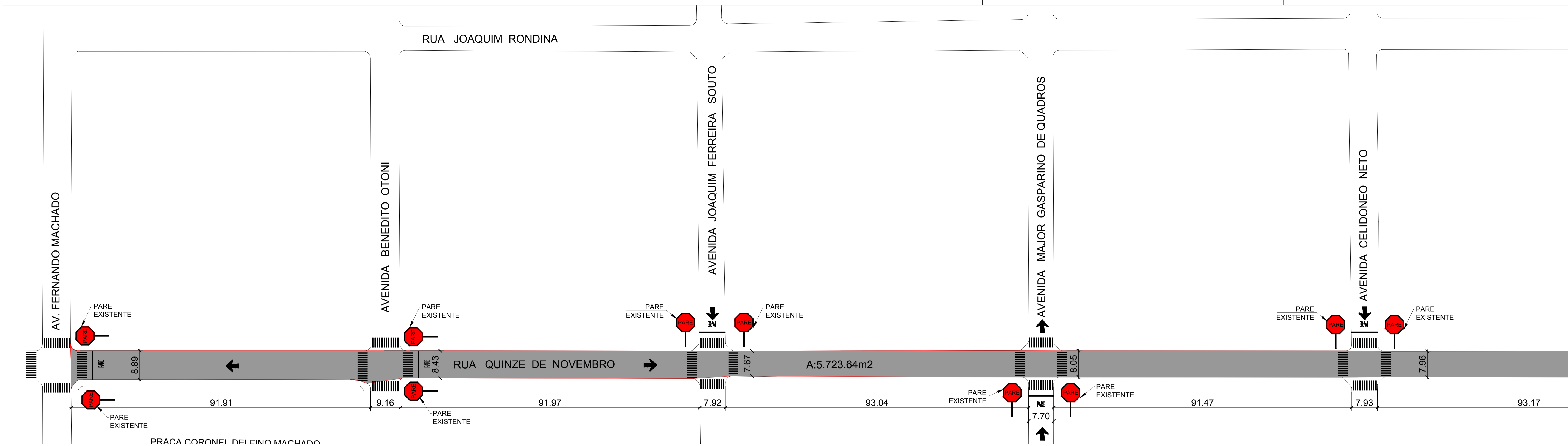
PLANTA - RECAPEAMENTO ASFÁLTICO E SINALIZAÇÃO DE TRÂNSITO ESCALA: 1:500
