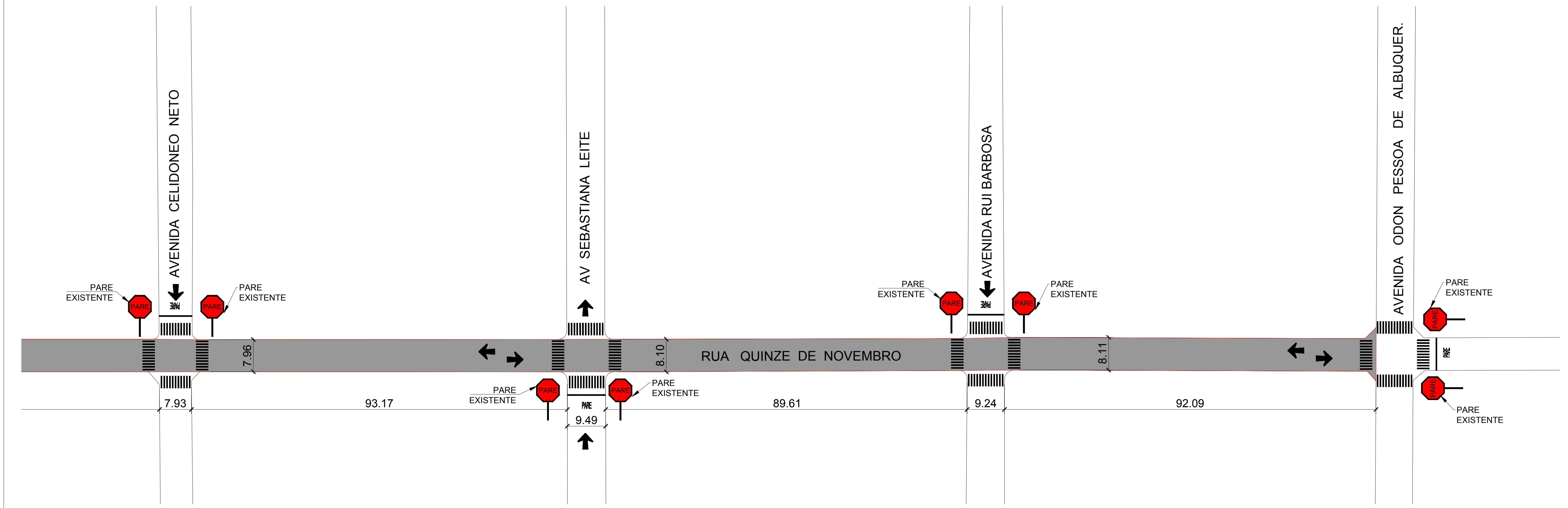
PLANTA - RECAPEAMENTO ASFÁLTICO E SINALIZAÇÃO DE TRÂNSITO ESCALA: 1:500
