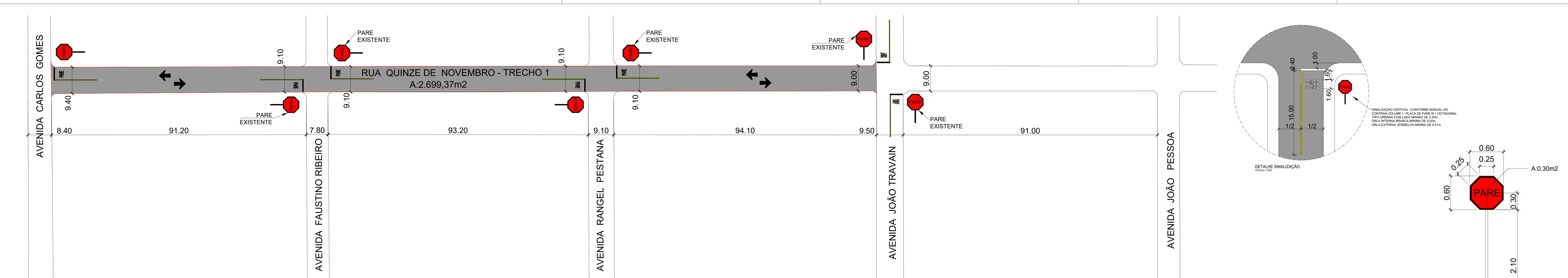
PLANTA - RECAPEAMENTO ASFÁLTICO E SINALIZAÇÃO DE TRÂNSITO - TRECHO 1 ESCALA: 1:500
