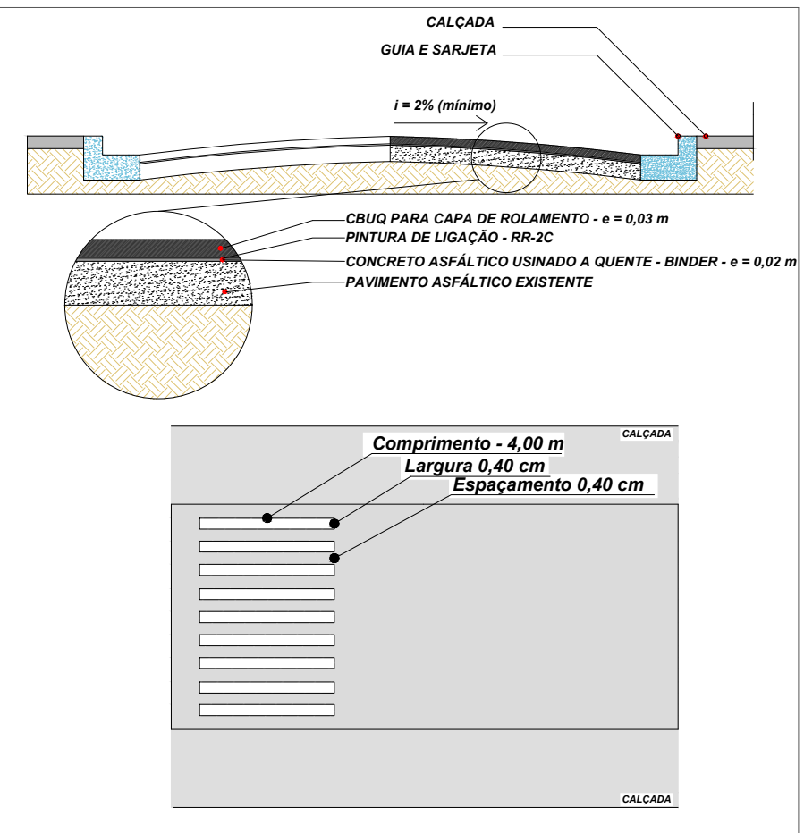
DETALHE CAMADAS DO RECAPE ASFÁLTICO E SINALIZAÇÃO HORIZONTAL Sem escala
