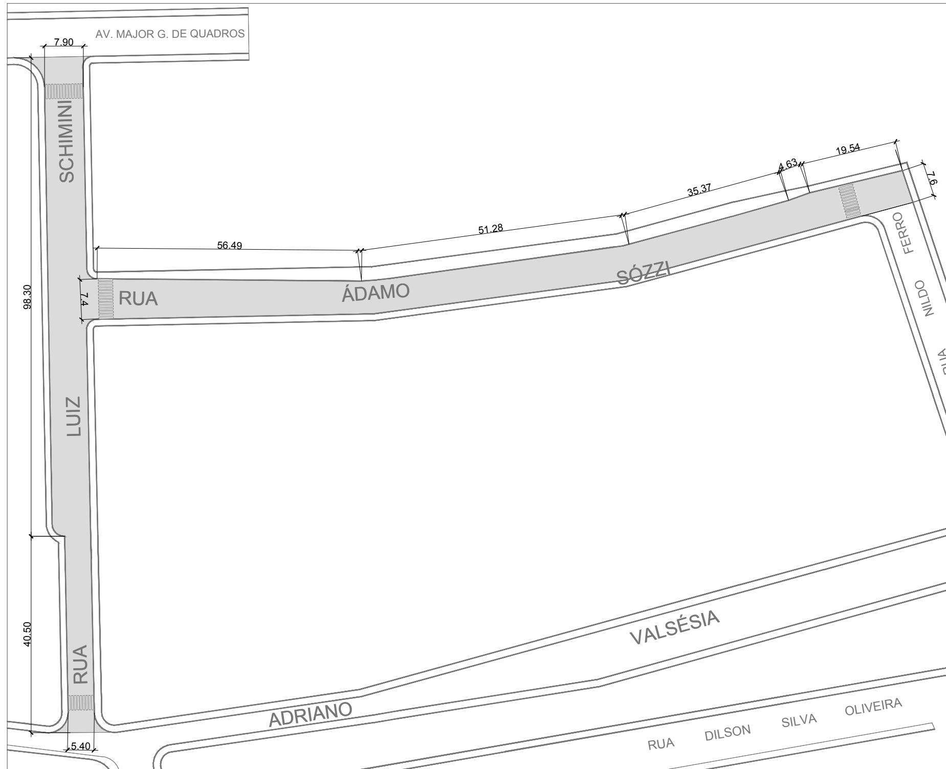
IMPLANTAÇÃO Sem escala
